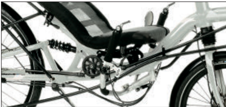
Komfortabel unterm Sitz. Arme und Nackenmuskulatur werden entlastet. Großer Einschlag durch indirekte Lenkung. Wartungsfreie Lagerung mit gedichteten Industrielagern und selbstschmierenden Gelenkköpfen.
